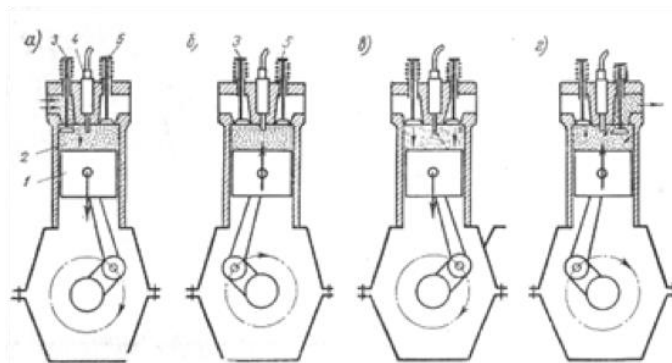
Рисунок 1- Рабочий процесс четырехтактного двигателя
